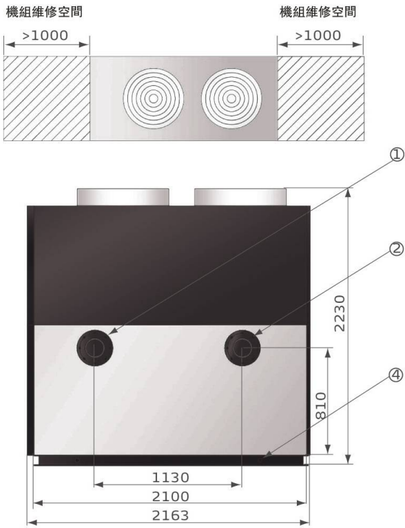
SICC-60A
