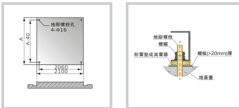
安裝基礎圖
