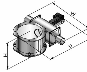
SBU-160-63S-V
