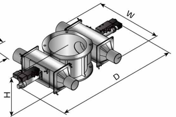
SBU-160-63D-V
