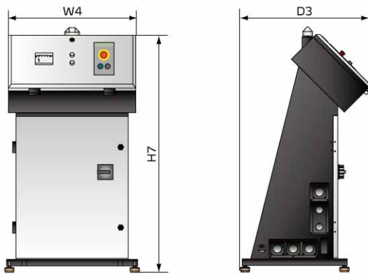
電控箱
