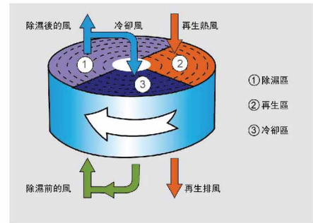
蜂巢轉輪示意圖
