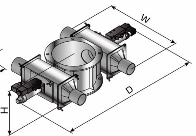
SBU-160-63D-V
