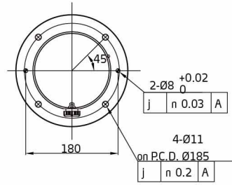
基座(俯視圖)
