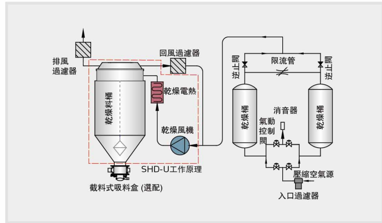
SHD-U-HD工作原理圖
