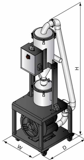
10HP (主機)
