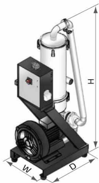
5HP (主機)
