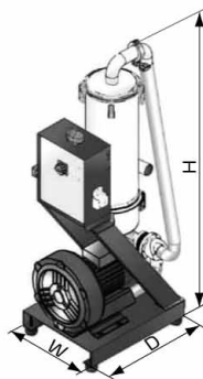
5HP (主機)
