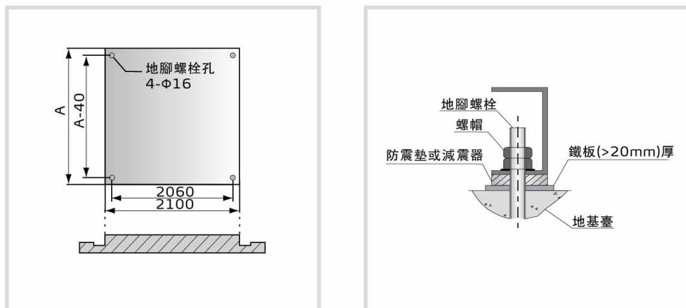
安裝基礎圖
