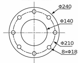
法蘭尺寸圖
