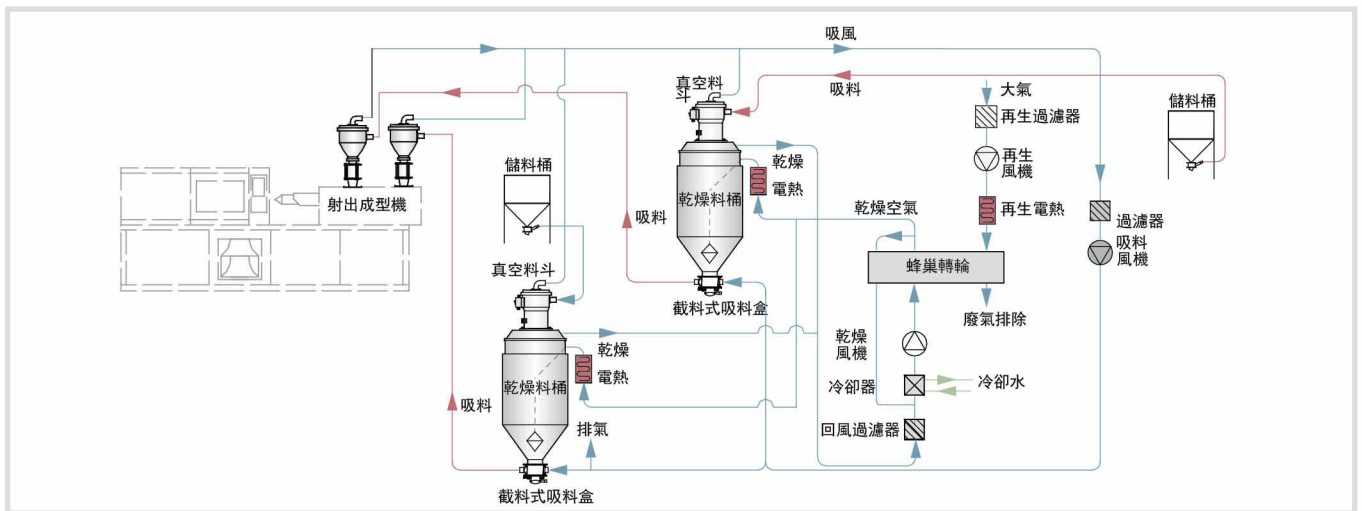
SCD-Ux2/H工作原理圖
