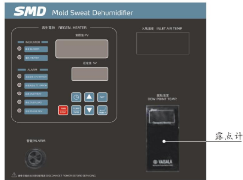
图 2-36: 嵌入式露点计图
