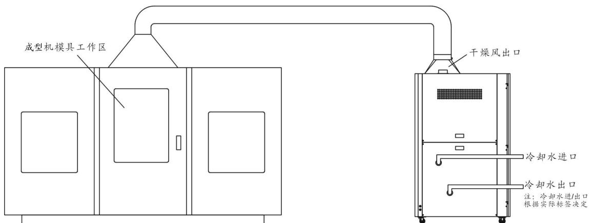
图 3-2: 水路连接示意图
